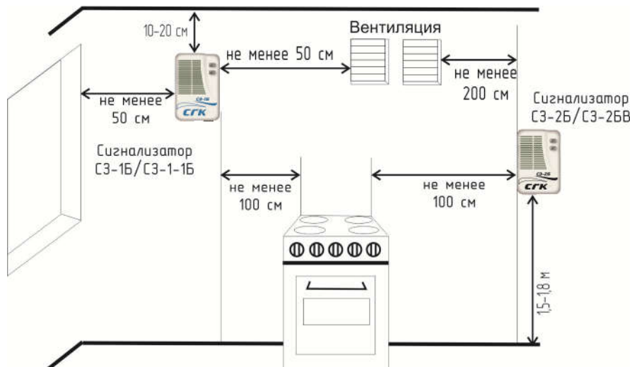
Рис.2 Схема размещения сигнализаторов загазованности SGK-C3.
